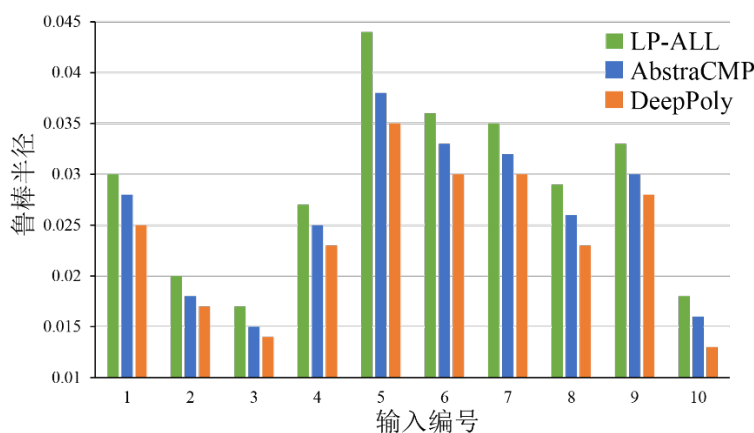
(b) MNIST 10 \times 80 网络的鲁棒半径对比
