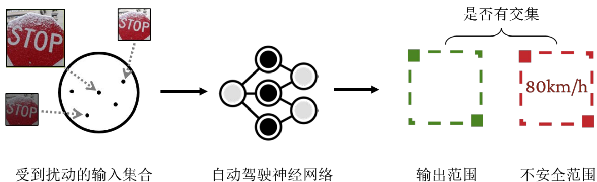
图 1-1 神经网络验证问题
