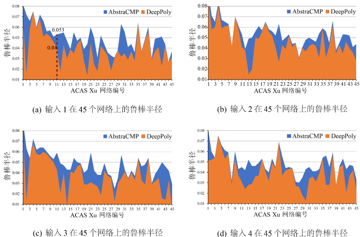
图 3-4 ACAS Xu 网络上能够验证的鲁棒半径对比
