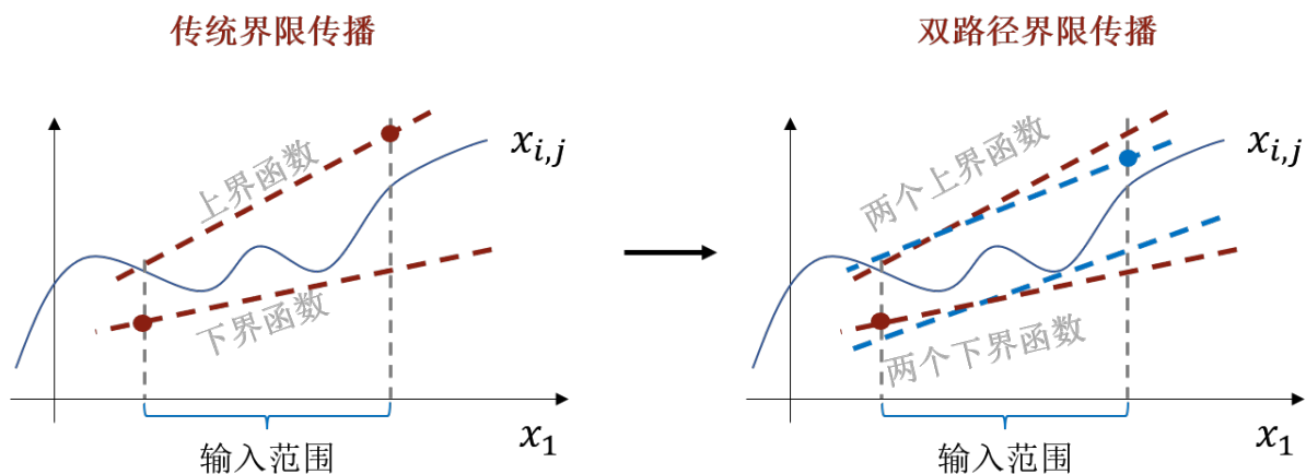
图 3-3 传统界限传播到双路径界限传播
