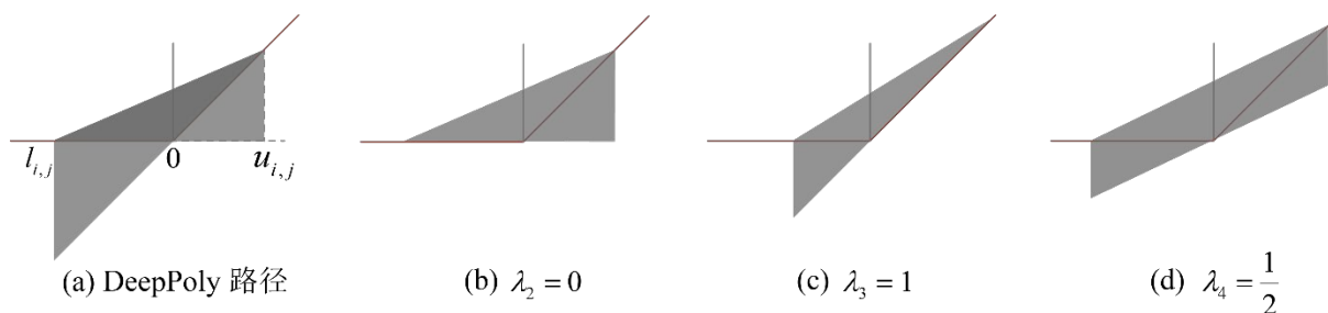
图 4-3 MpBP 默认使用的四条界限传播路径
