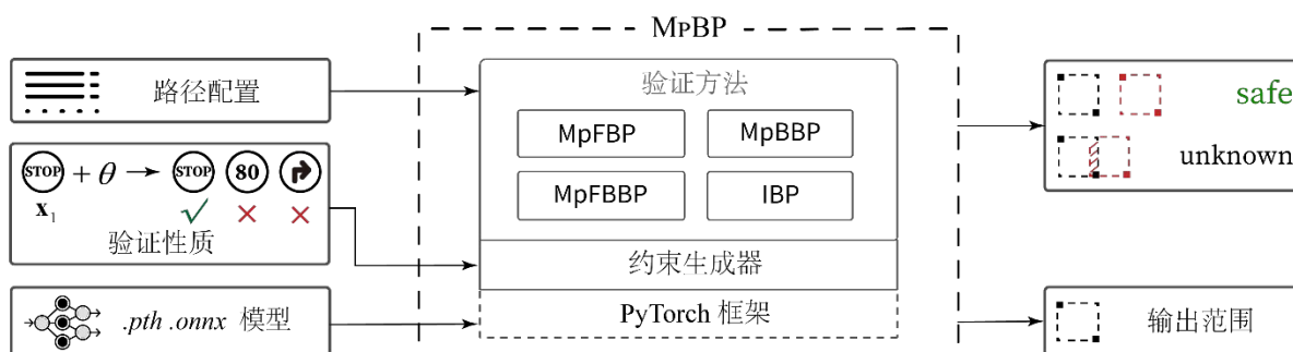
图 4-2 工具 MpBP 的框架
